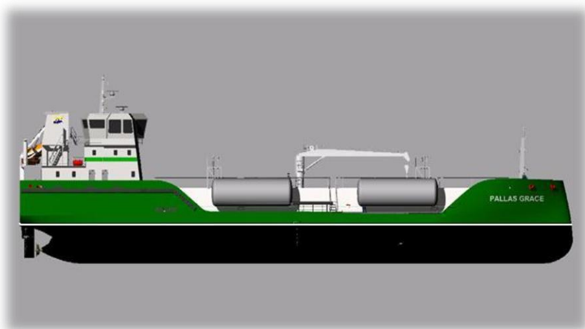
Pallas nya koncept för ett framtidens miljö-bunkringsfartyg går under namnet Pallas Grace.
