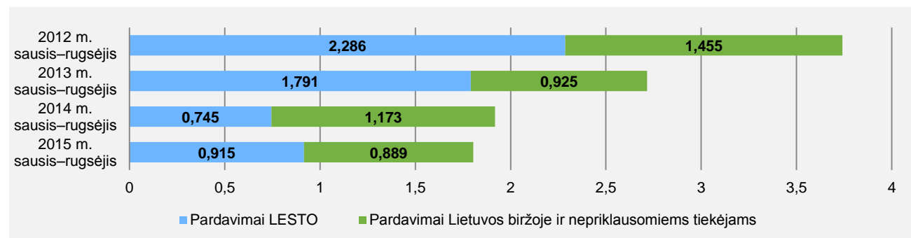
Bendrovės elektros energijos pardavimai vidaus rinkoje (TWh)
