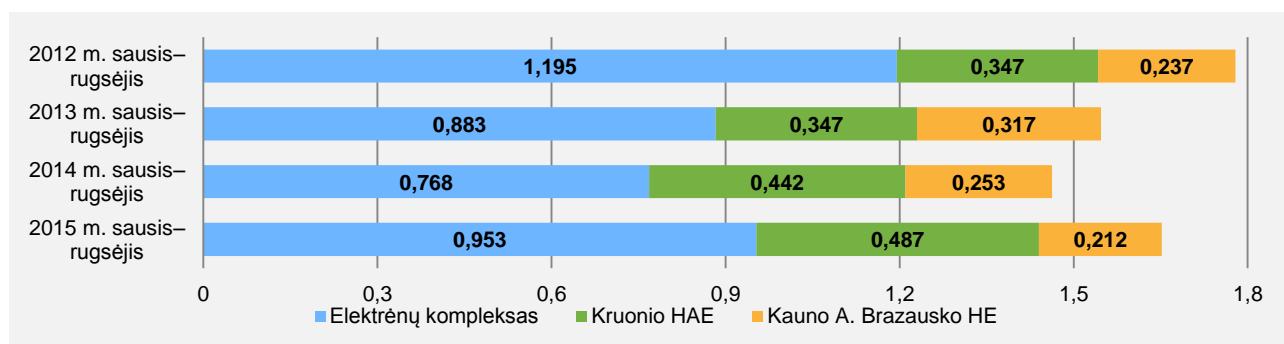
Bendrovės valdomose elektrinėse pagaminta ir parduota elektros energija (TWh)
